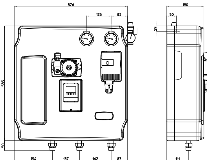
Figura 3: dimensioni d'ingombro ed interessi significativi del modulo
